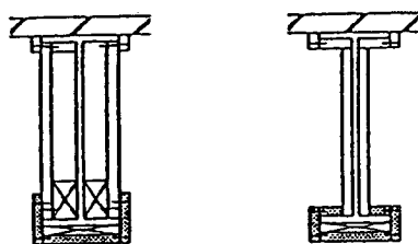
垂直断面図
