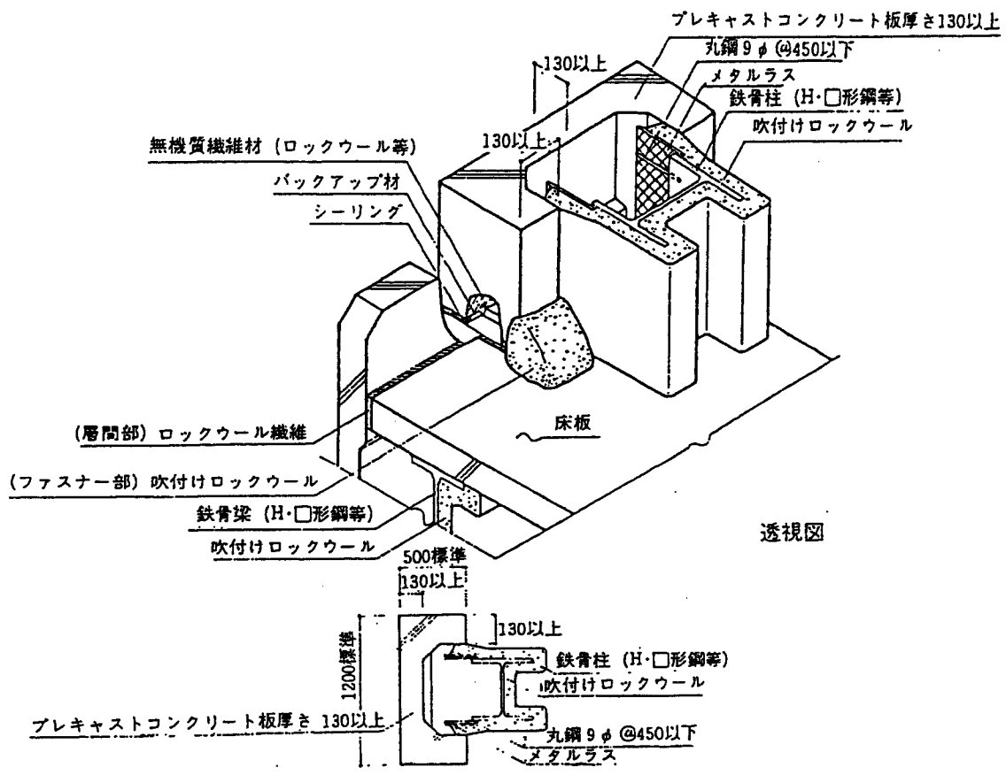
断面図1 メタルラス下地構成の場合
