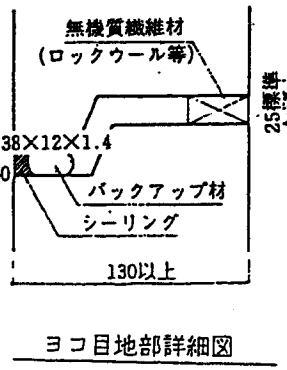
断面図2 鉄板 (厚さ0.4以上) 下地構成の場合
